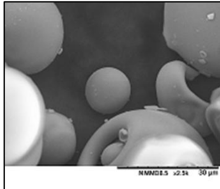
図. SEM×2500
